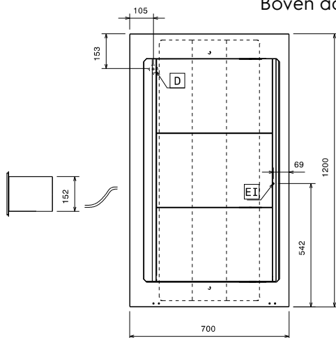
Boven aanzicht
