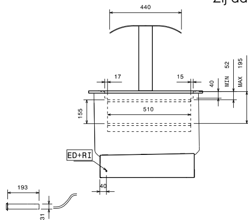
Zij aanzicht
