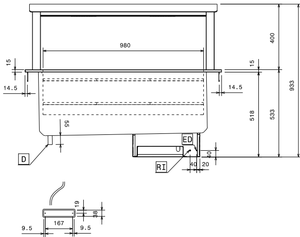
Front aanzicht
